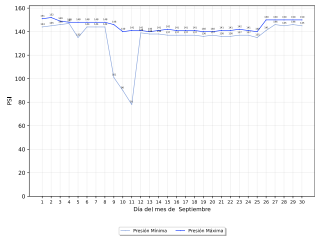
Comportamiento de presión de sistema
