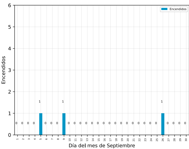
Conteo de arranques de bomba jockey
